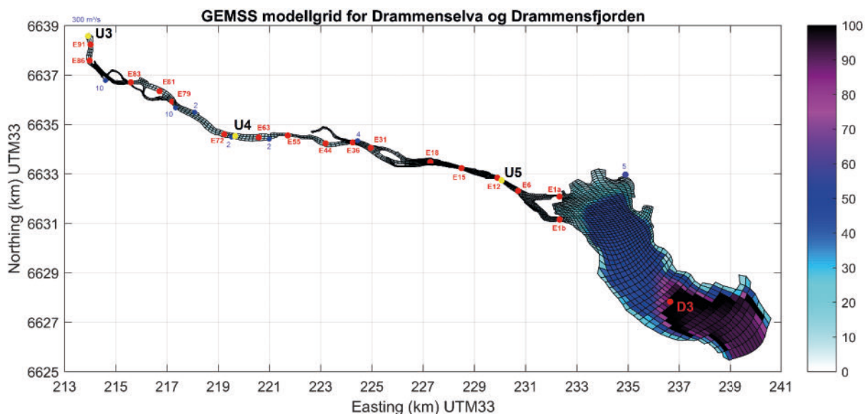
Figur 6. Modellens rutenett hvor fargeskalaen angir vanddybden i meter. Ved Hellefoss er det lagt inn en vannføring på 300 m 3 /s. De blå punktene med et blått tall, angir tilløp til Drammenselva hvor tallet angir vannføring i m 3 /s. De tre utslippspunktene U3 til U5 er markert med gule punkter. De røde punktene er stasjoner hvor det er tatt ut data fra modellen.
