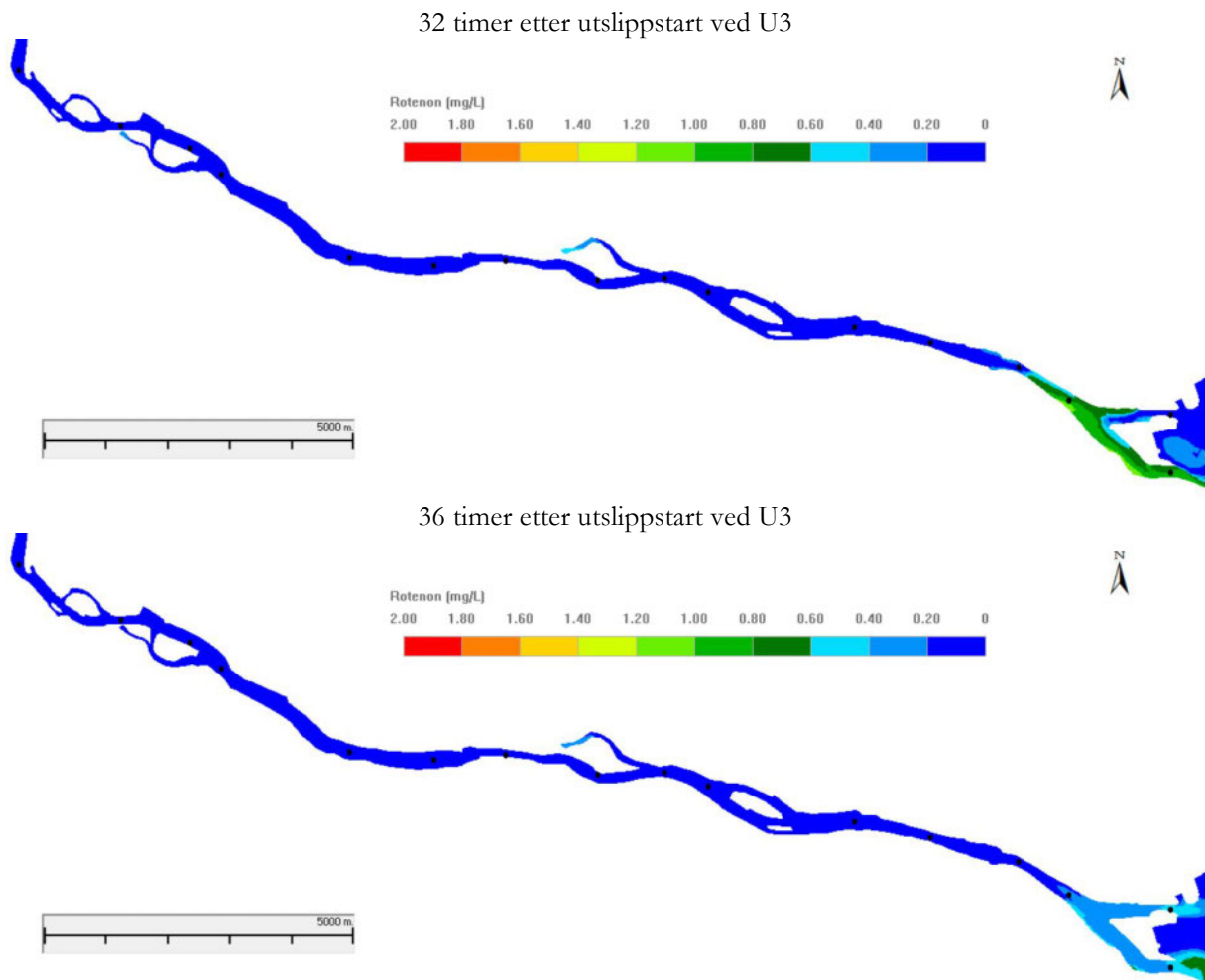
Figur 12. Konsentrasjon av rotenonløsning (mg/L) i Drømmenselvas overflatelag ved to tidspunkter.
