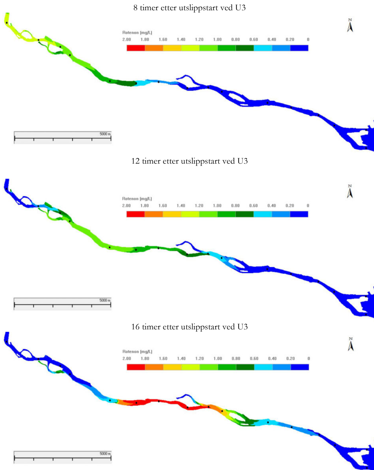
Figur 10. Konsentrasjon av rotenonløsning (mg/L) i Drammenselvas overflatelag ved tre tidspunkter.
